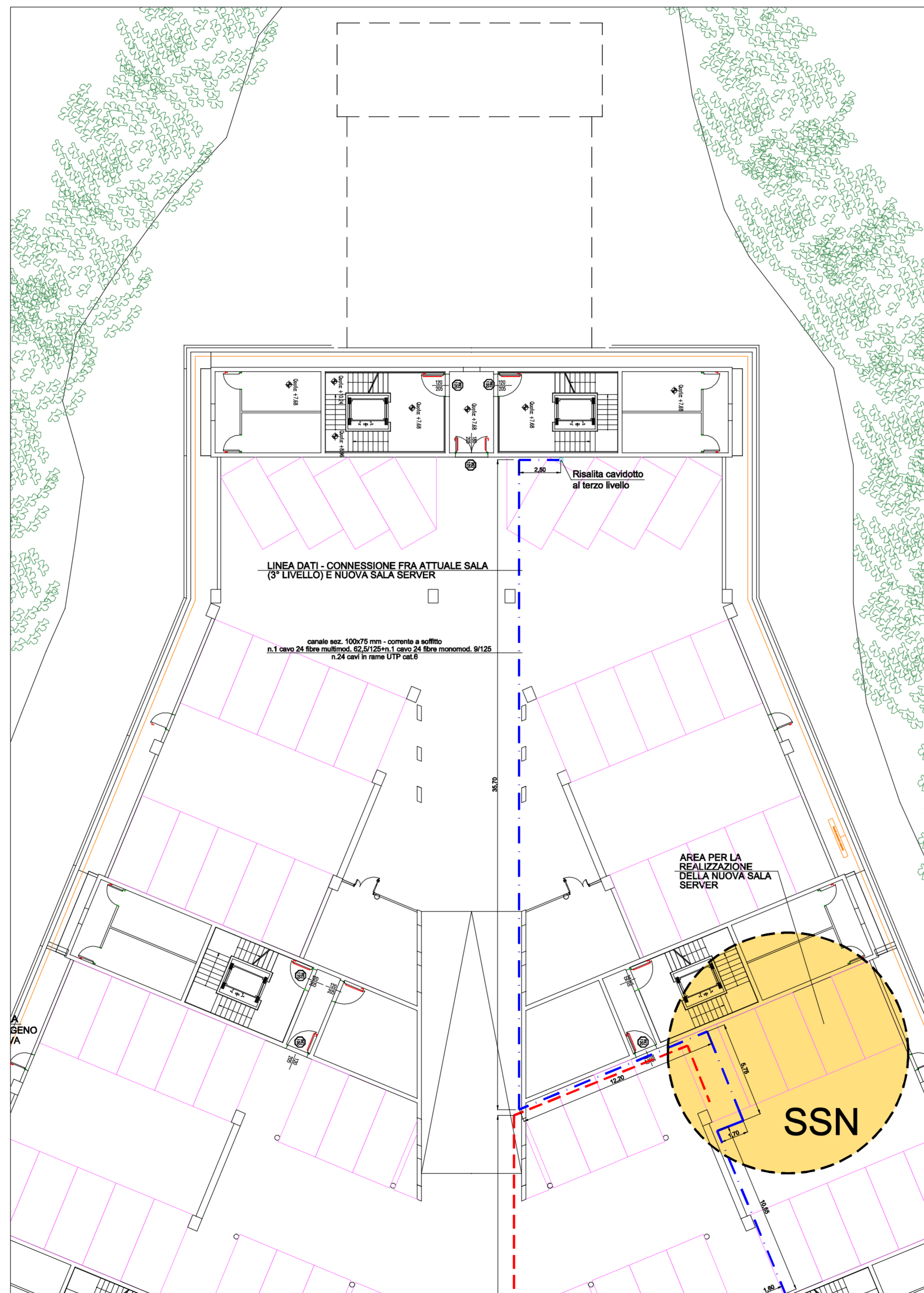
PIANO INTERRATO GARAGE - 1° LIVELLO [1:100]
