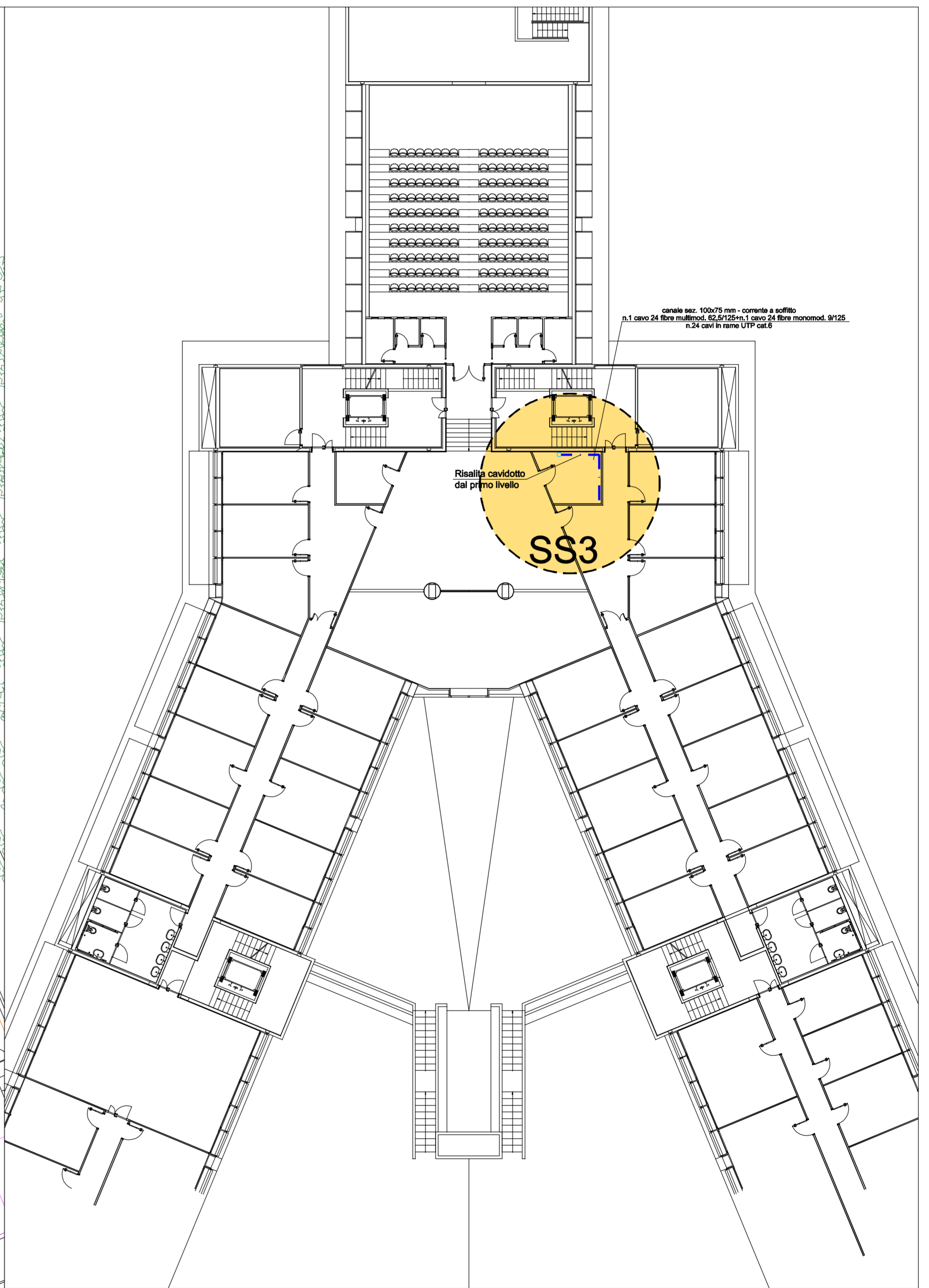
PIANO PRIMO - 3° LIVELLO [1:100]
