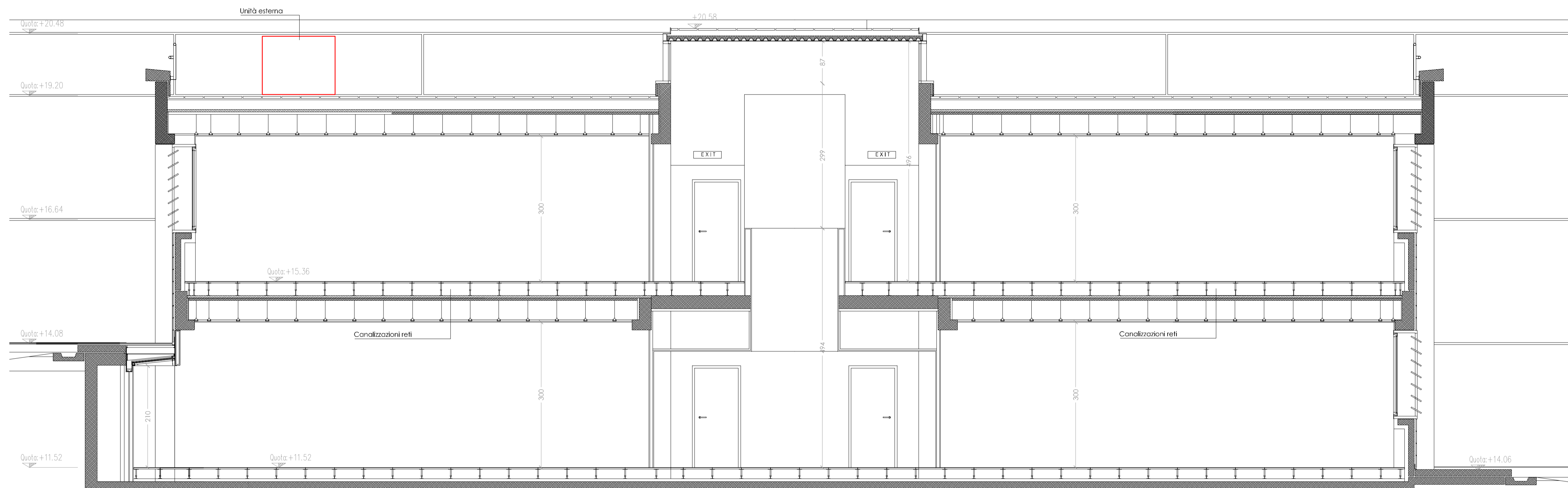
SEZIONE SU LABORATORI
