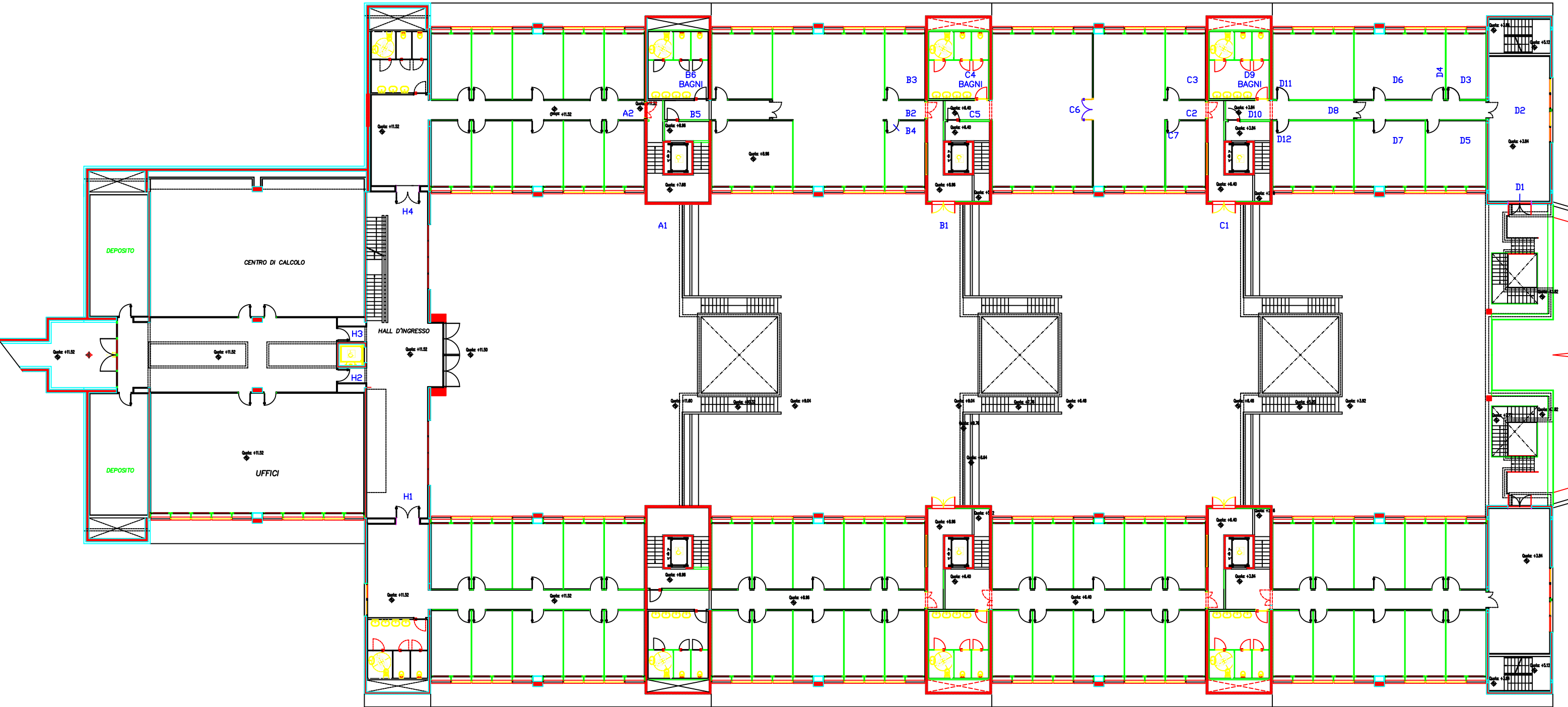
EDIFICIO 1 Pianta piano terra
