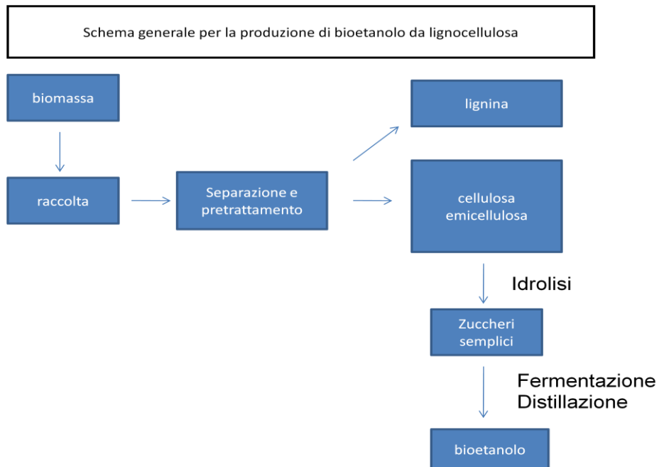
Figura 3.12 - Produzione di bioetanolo da lignocellulosa.
