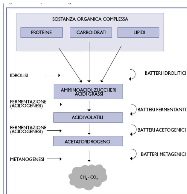
Figura 4.1 - Fasi del processo di digestione anaerobica (fonte CETA).
