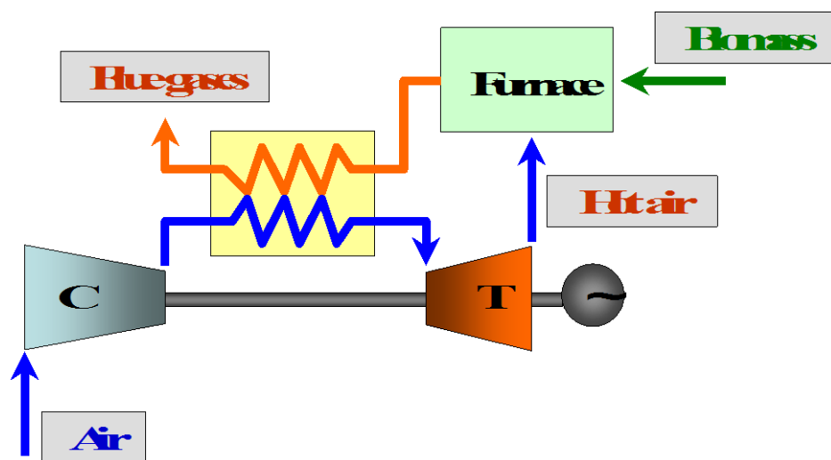
Figura 2.6 - Impianto EFGT.
