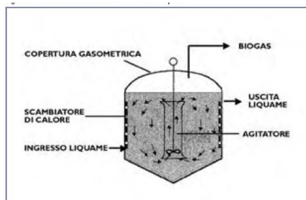
Figura 4.3 - Schema di reattore a miscelazione completa (fonte CETA).
