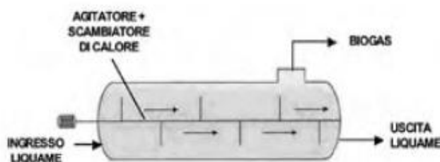
Figura 4.4 - Schema di reattore con flusso a pistone (fonte CETA).
