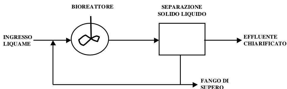
Figura 4.5 - Schema di reattore biologico con ricircolo.
