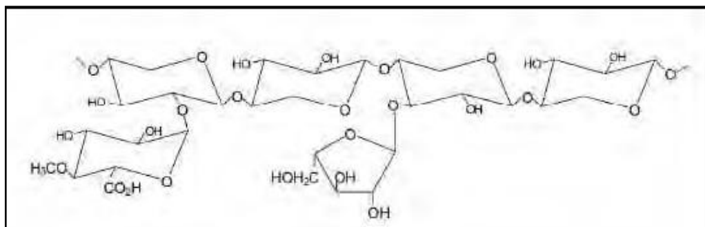
Figura 3.13 - Struttura dell'emicellulosa
