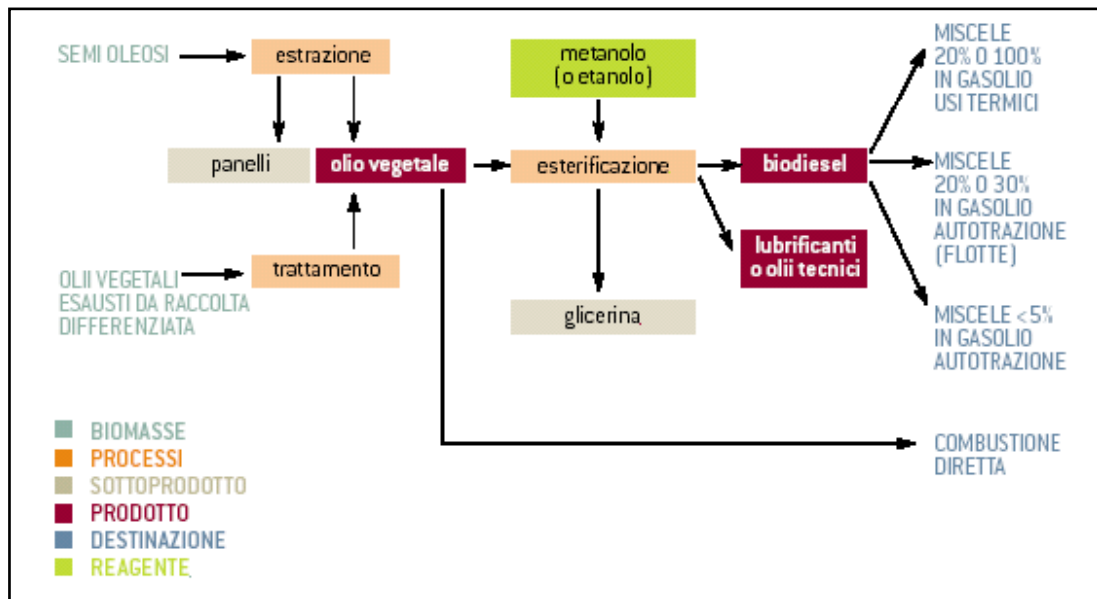
Figura 3.3 - Schema di produzione del Biodiesel.
